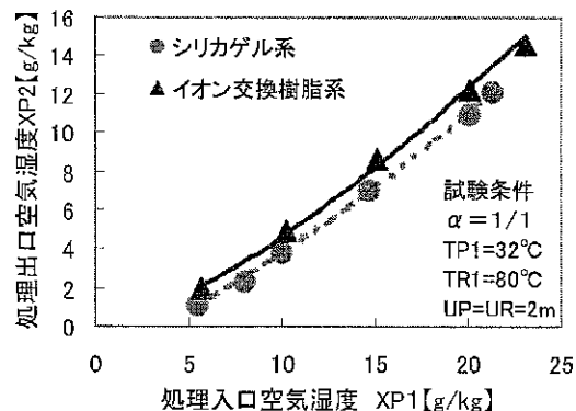
図2 除湿性能比較図
