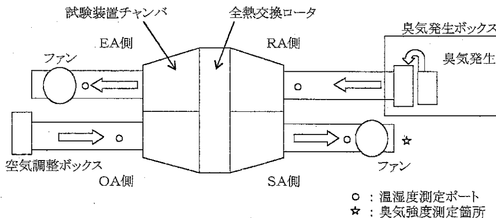
図1 試験装置図
