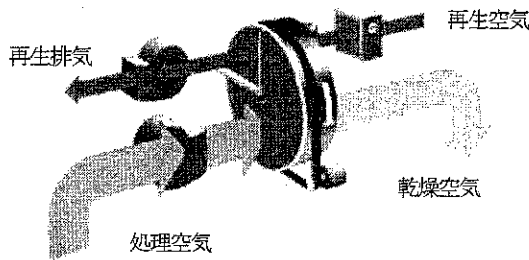
図1 産業用デシカント除湿機フロー
