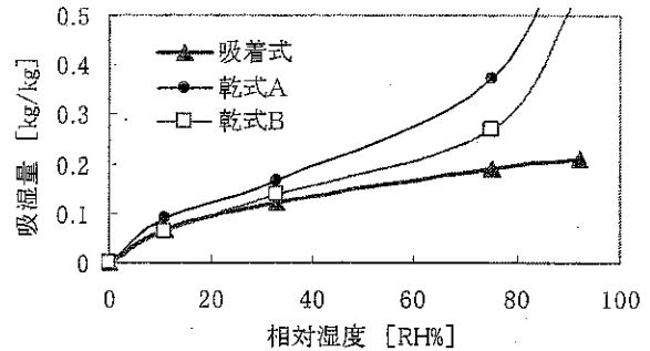
図2 平衡吸湿量の比較
