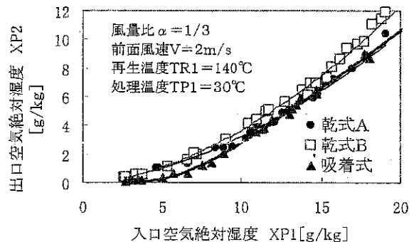
図3 除湿性能比較
