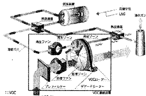
図1 VOC濃縮燃焼フロー
